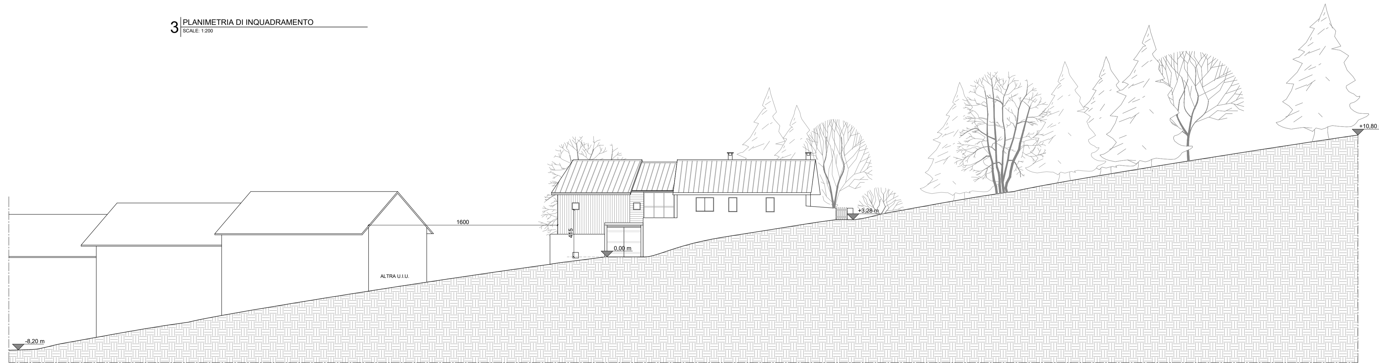
4 SEZIONE TERRITORIALE AA SCALE: 1:200
