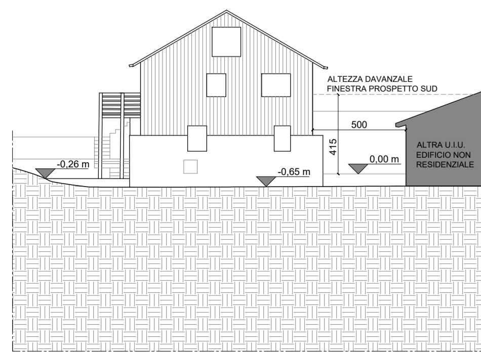
2 SEZIONE TERRITORIALE BB SCALE: 1:200
